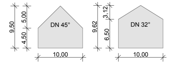
Skizze Firsthöhe
